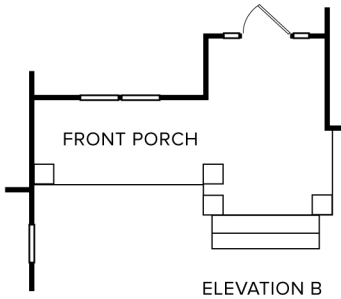
ELEVATION B
